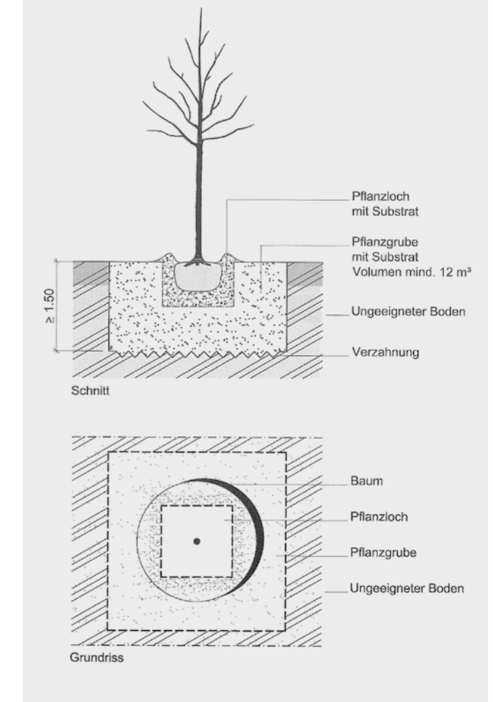
Abb. 38: 2 FLL Pflanzgruben-Skizzen
